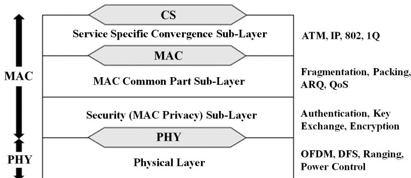
Fig. 1.20. IEEE 802.16 layers.
